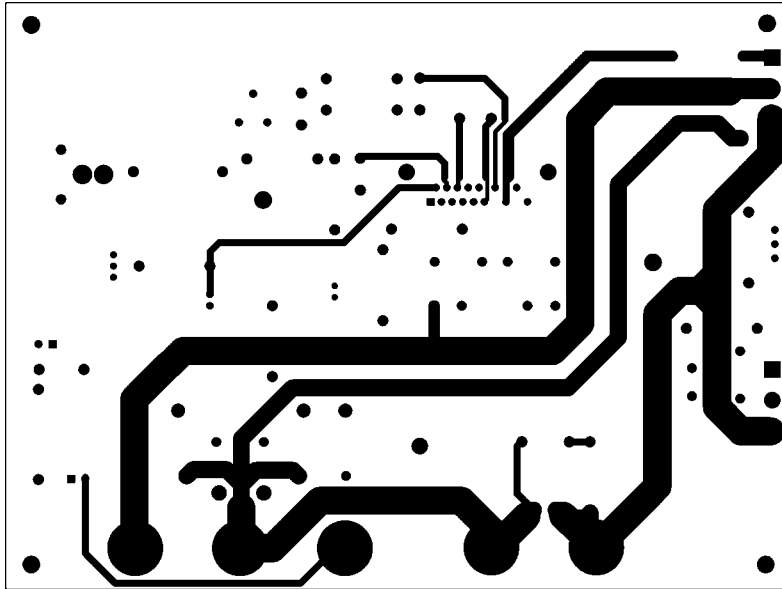
Bottom Layer
