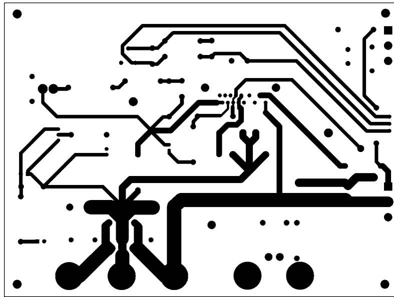
Top Layer
